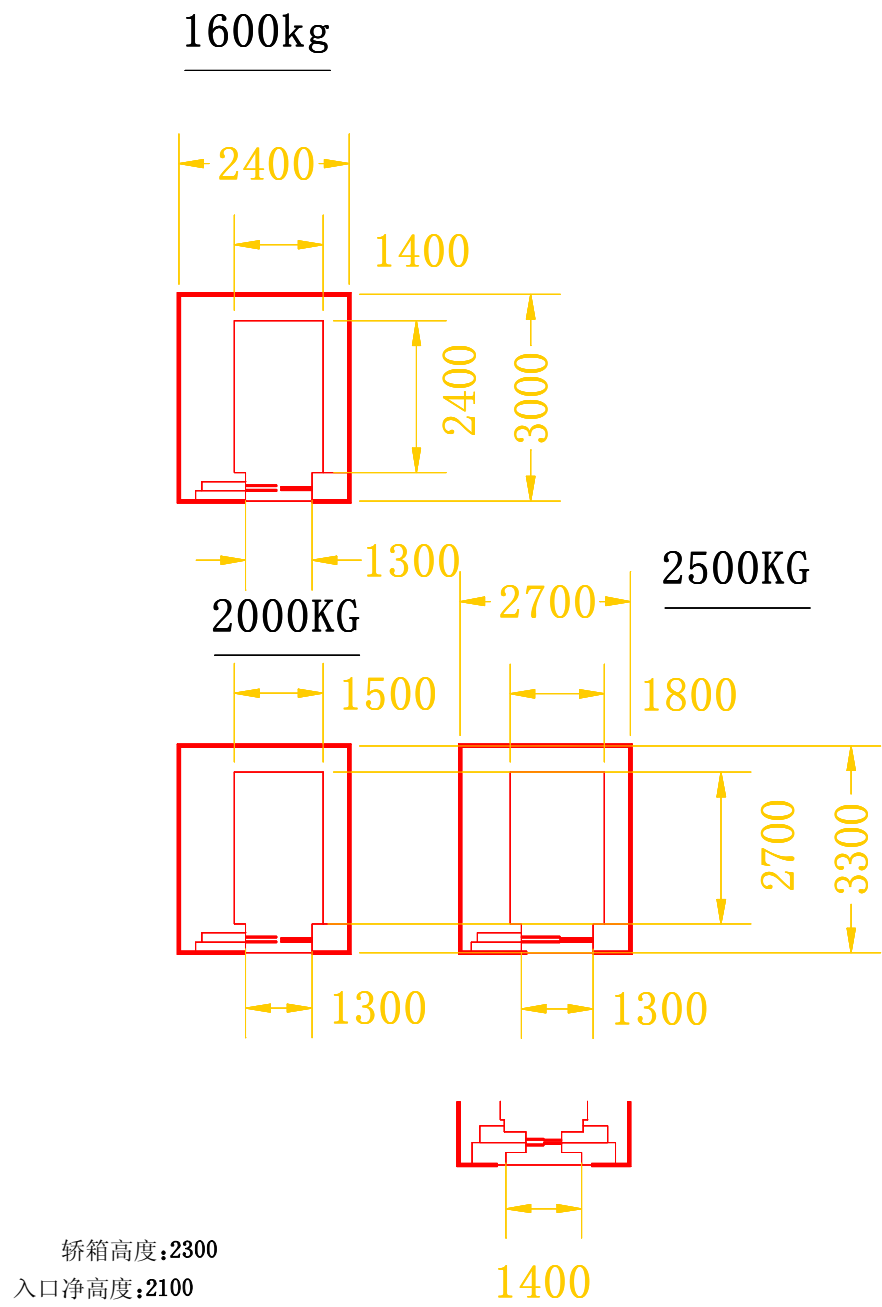
图 4 病床电梯井道平面图
